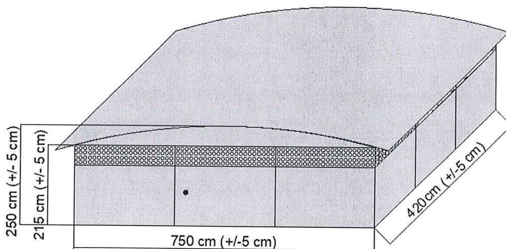
RYСУNEK POGŁĄDOWY- WIATA ŚMIETNIKOWA Z WEJŚCIEM PO DŁUŻSZEJ KRAWĘDZI
